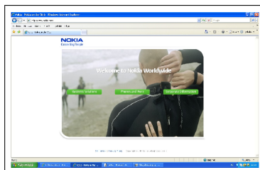
Kuva 31: Kohdeasiakkaan kotisivu.
