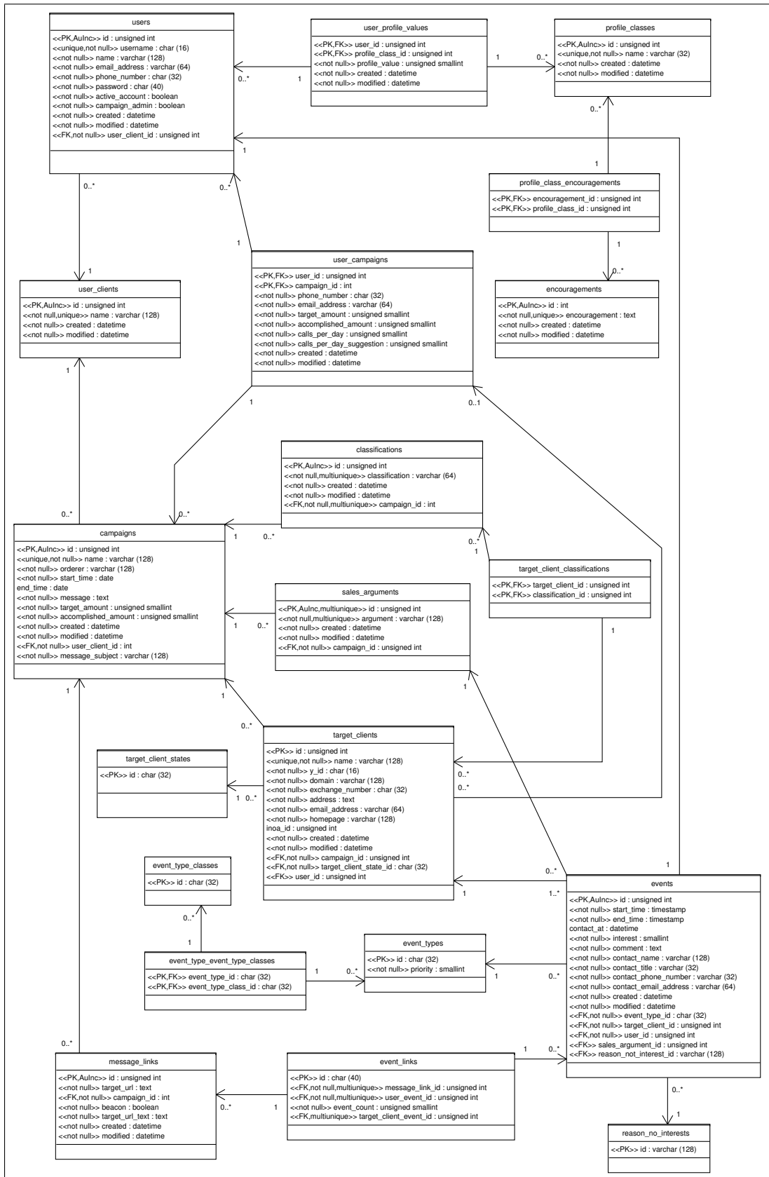
Kuva 2: Tietokantakaavio.
