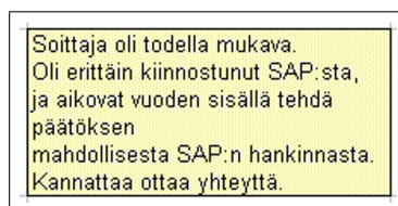
Kuva 30: Kommentti.
