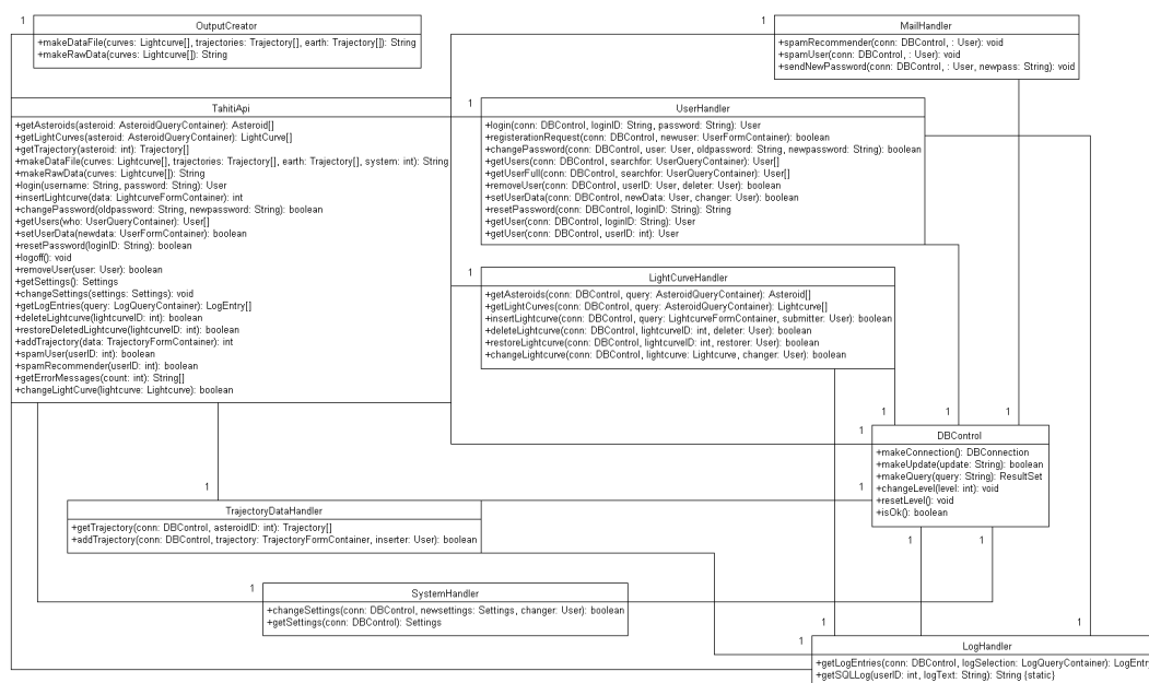
Kuva 4: Järjestelmän luokkakaavio
