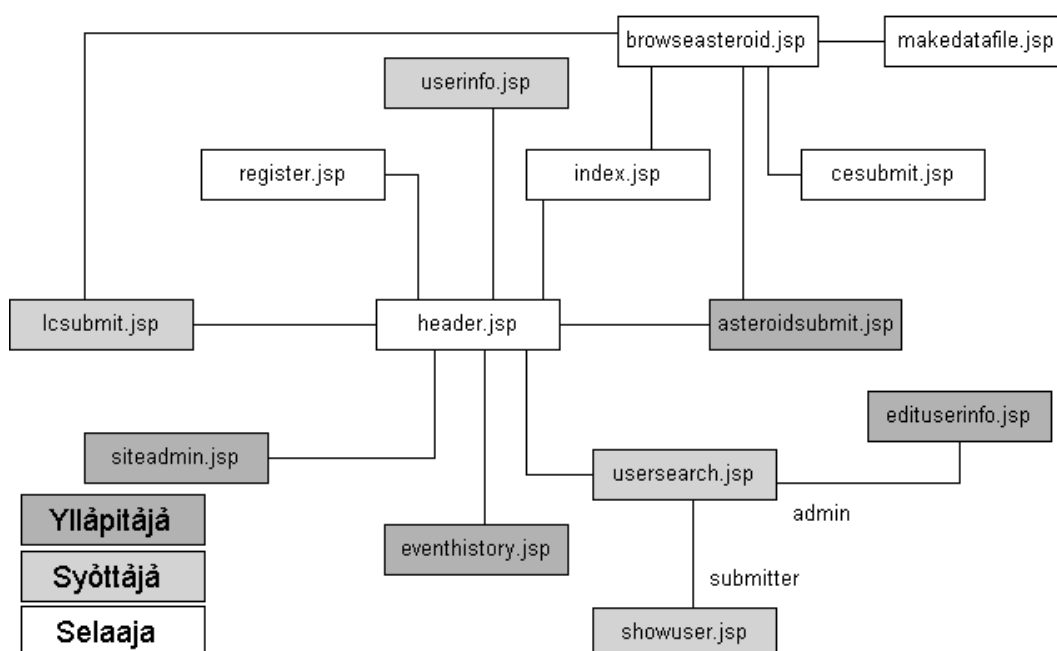
Kuva 15: Järjestelmän sivukartta.
