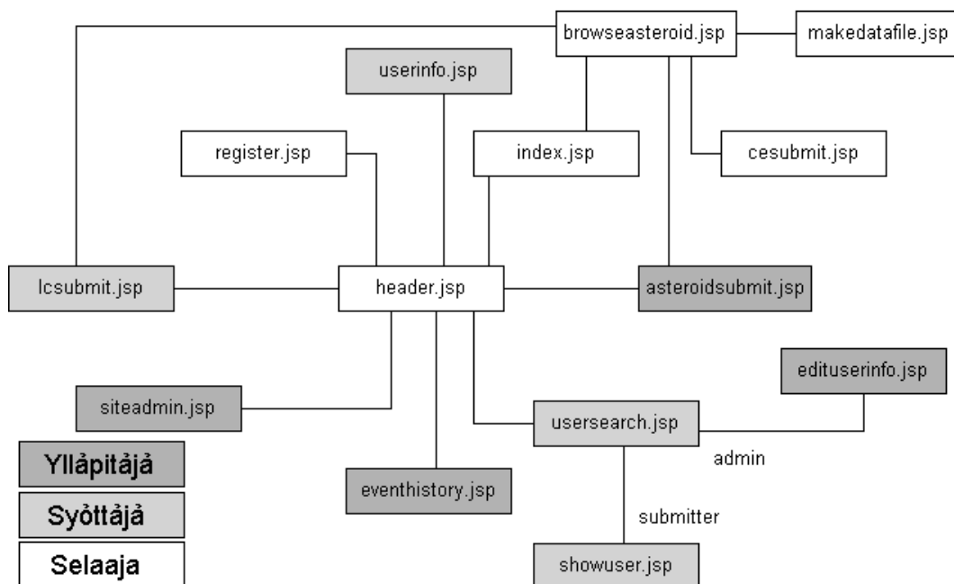
Kuva 15: Järjestelmän sivukartta.
