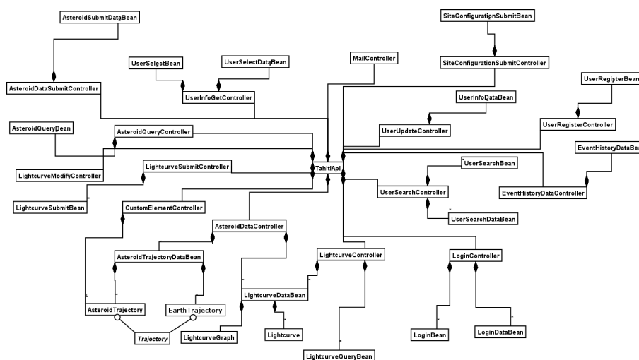
Kuva 13: Käyttöliittymäluokkien luokkakaavio
