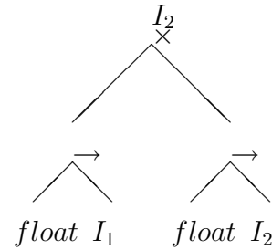
Kuva 2: Rekursiivisia rajapintarakenteita
