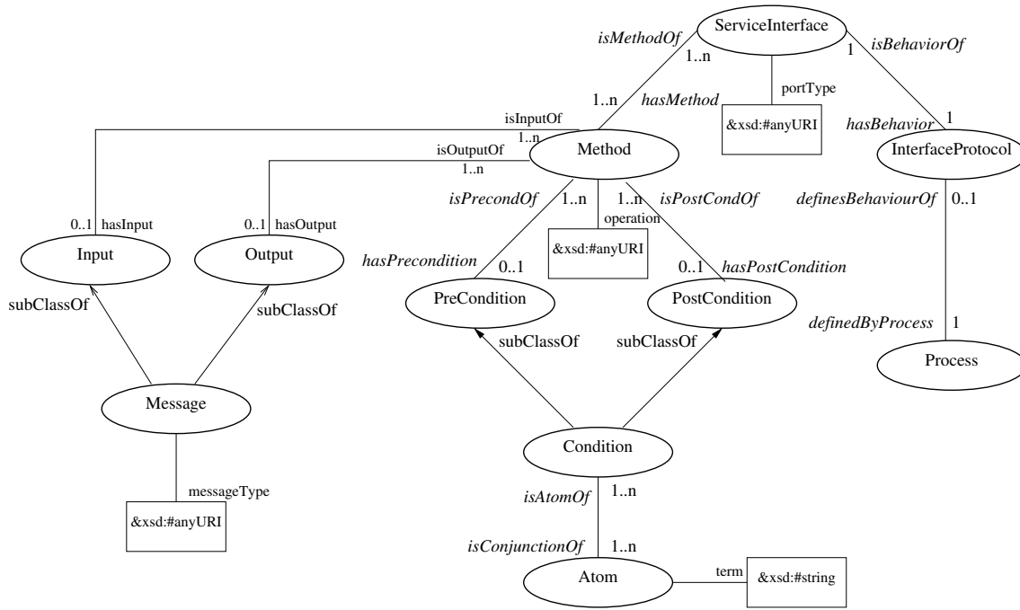
Kuva 21: ServiceInterface-ontologian rakenne
