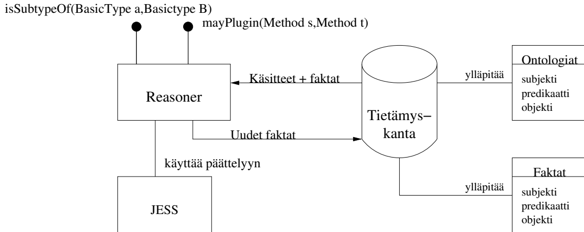
Kuva 23: Reasoner-komponentin yleiskuva
