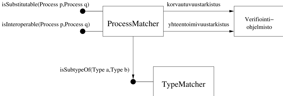
Kuva 24: ProcessMatcher-komponentin yleiskuva
