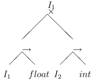
Kuva 2: Rekursiivisia rajapintarakenteita
