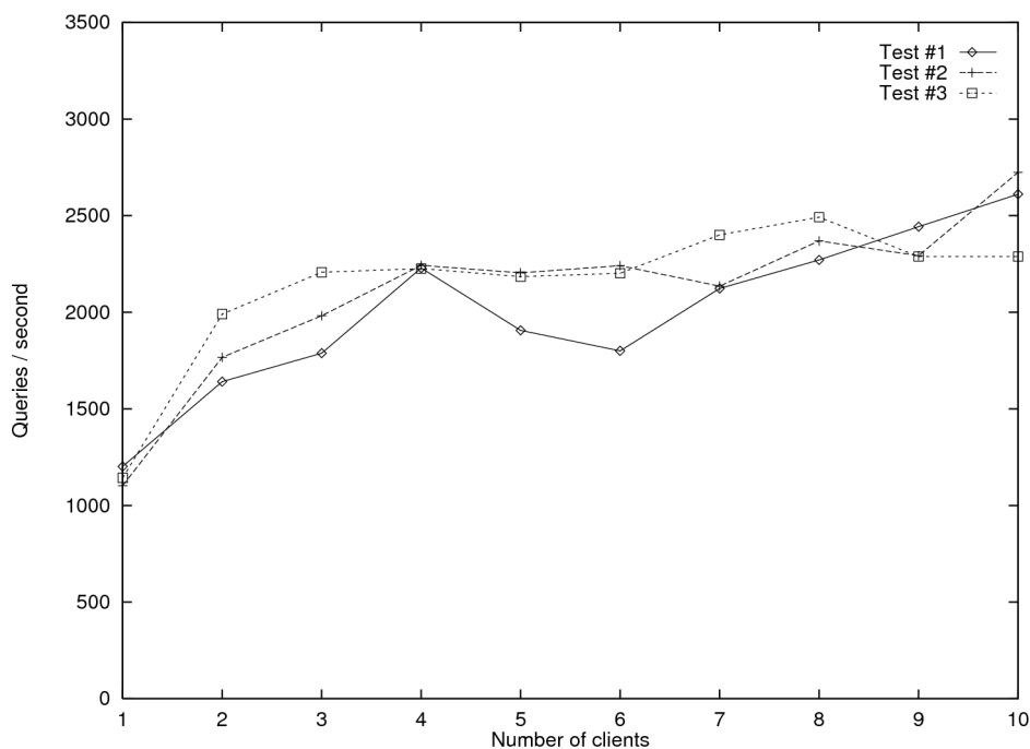
Kuva 1: Kuvan elementit.
