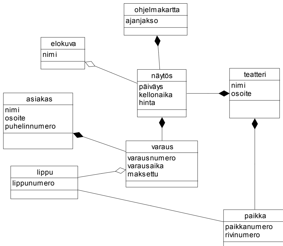
Kuva 4.32: Luokkakaavion seuraava versio
