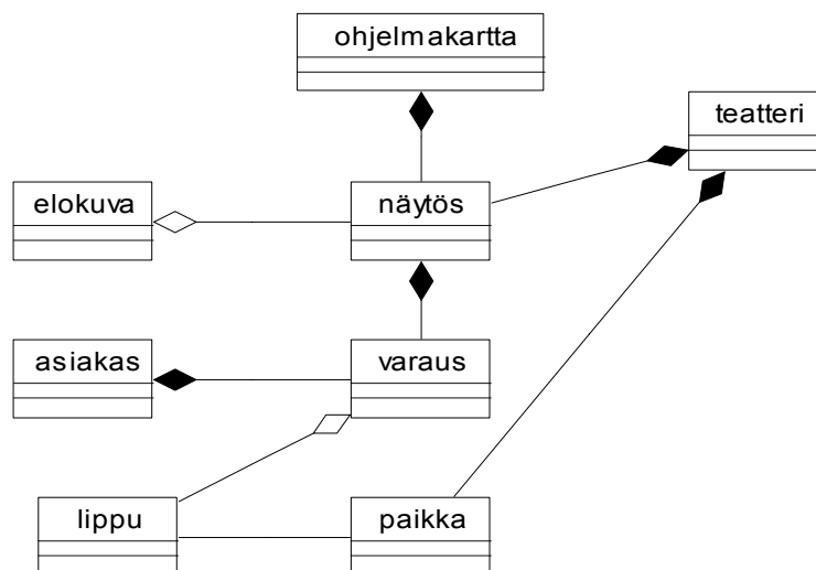
Kuva 4.31: Luokkakaavion seuraava versio.
