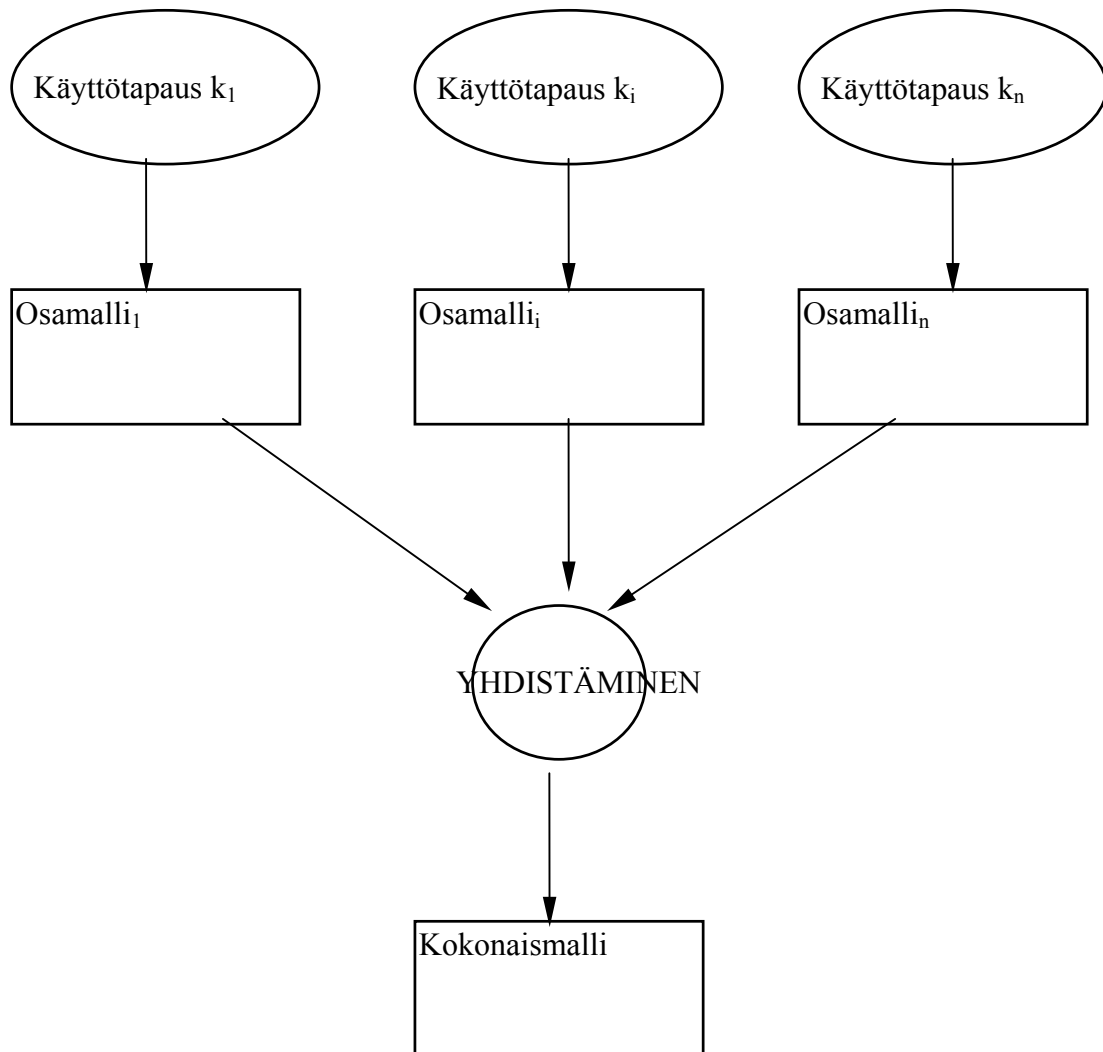
Kuva 4.33: Käyttötapauspohjainen tietosisällön määrittely
