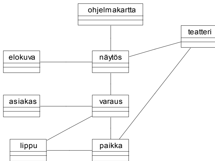
Kuva 4.30: Luokkakaavion ensimmäinen luonnos.
