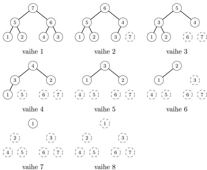
Kuva 7.5: Esimerkki kekojärjestämisestä.
