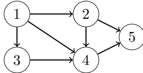
Kuva 10.6: Suunnattu verkko.
