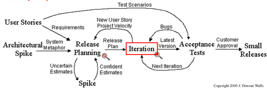
Kuva 1: XP:n prosessi [2]
