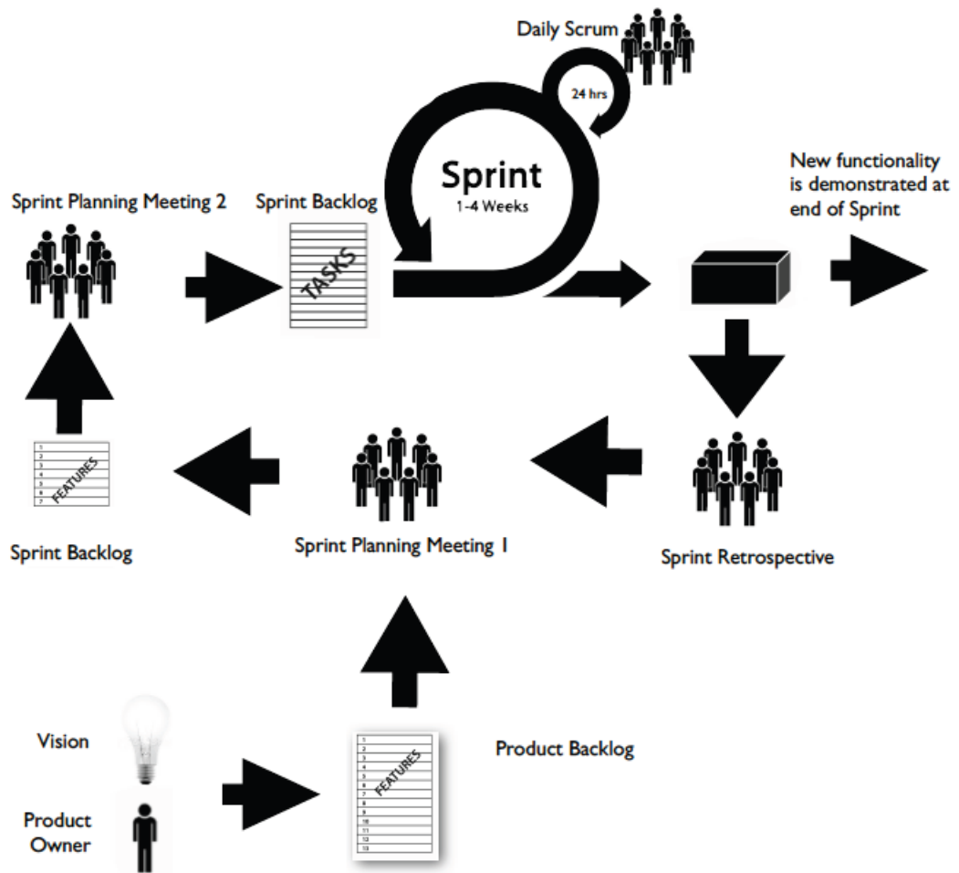
Kuva 2: Scrumin prosessi [24]
